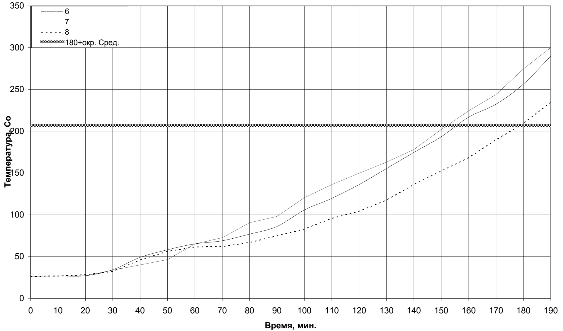
Рис. 8. Изменение температуры образца №2 при испытании
